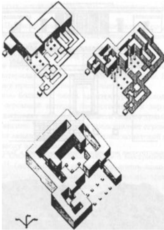
Ил. 65. Реконструкция плана храма Окса в Тахти Сангине
