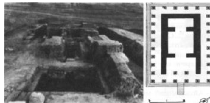
Ил. 61. Вид и план периптерального мавзолея в Ай Ханум
