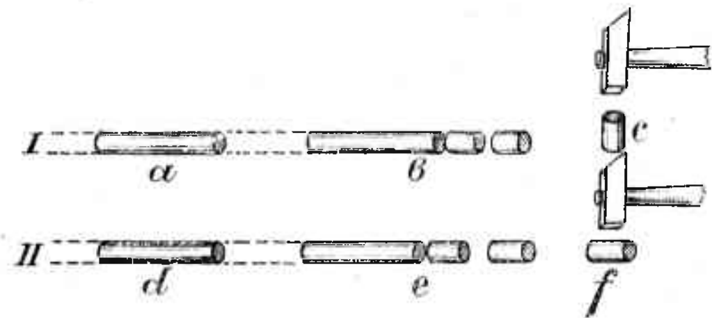
Табл. 62. Техника изготовления монетных кружков.
