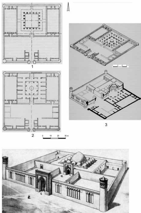
Рис. 10. Рабат-и Малик: 1 – план I периода; 2 – план II периода; 3 – аксонометрия II периода; 4 – реконструкция II периода (по Н.Б. Немцевой)
