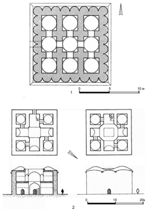
Рис. 23. Закрытые здания: 1 - Ат-Тахмаладж, X–XI вв. (по Г.А. Пугаченковой); 2 – Зиндан-и Харун ал-Рашид, X–XI вв. (по В. Кляйссу)
